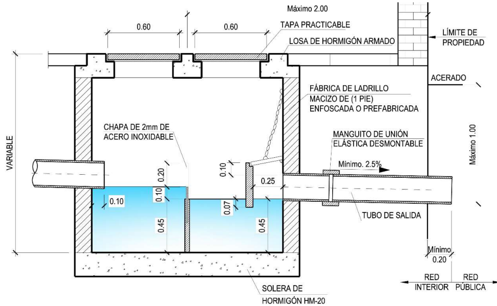
ALZADO-SECCIÓN
