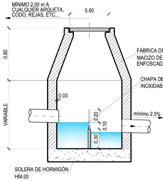
ALZADO-SECCIÓN
